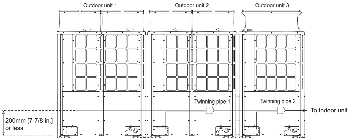
<PUHY-EP950, 1000, 1050YSNW-A>
